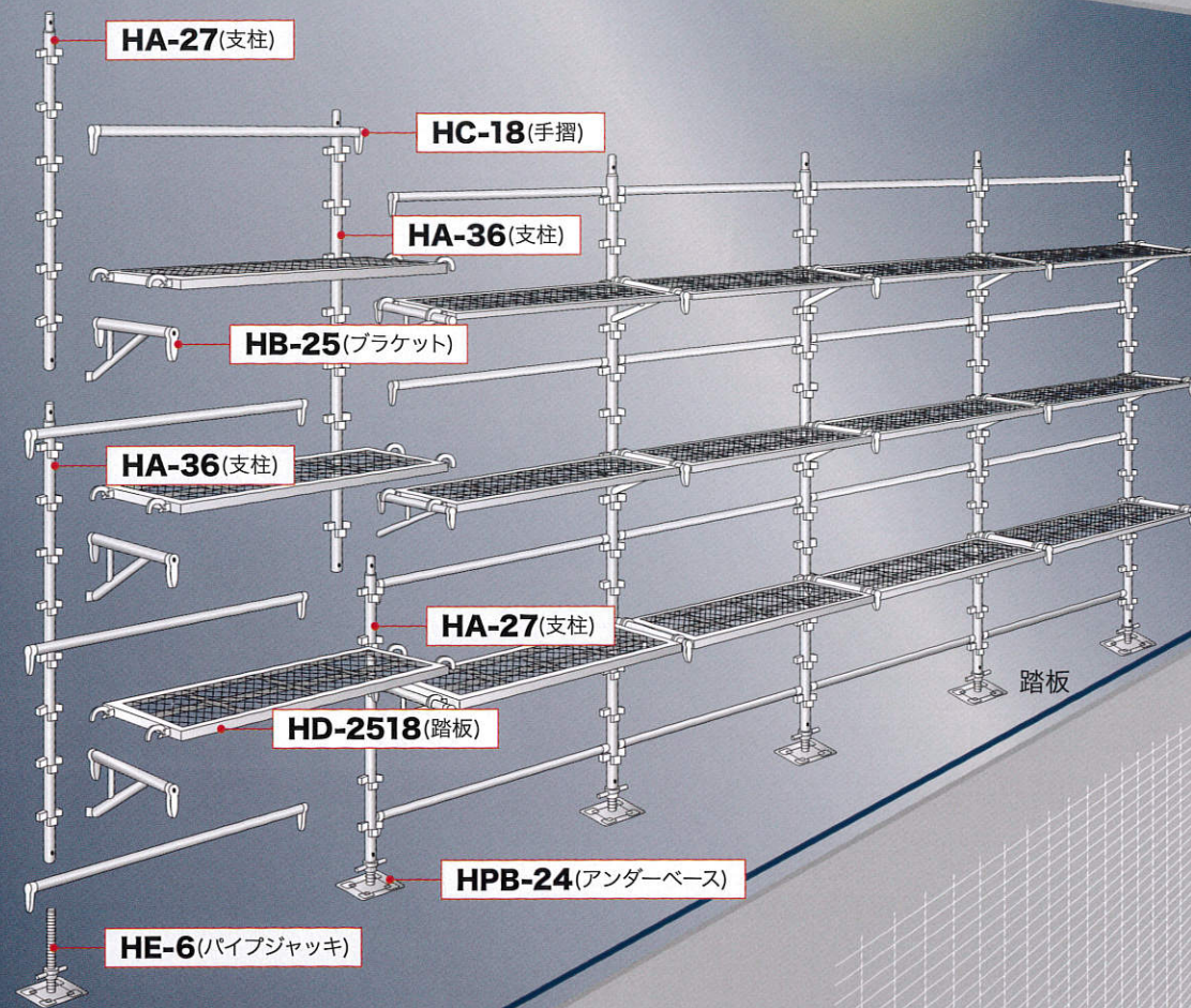
ヘイワビルダー組立図(3層×5スパン使用例)
